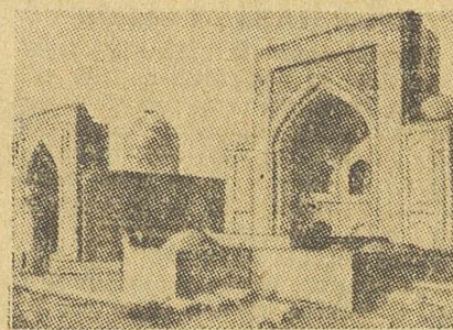
Meczet w rejonie Buchary ocalał dzięki zastosowaniu „poduszki” trzciny w cokole budowli.
