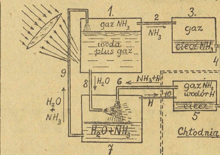
Uproszczony schemat chłodziń absorpcyjnej (amoniakalnej). Opis w tekście.
